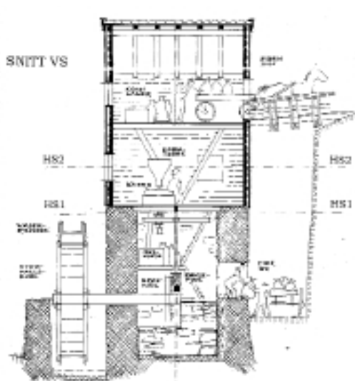
(Figurtekst tegning 1:) Ellingsrud mølle fra 1795. Et vertikalt snitt innvendig med to horisontale snitt. Tegnet av Bjørn Berge.
