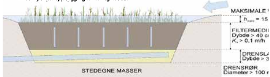
Eksempel på oppbygging av et regnbedd.
